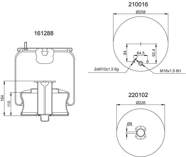
(Steel Piston)
